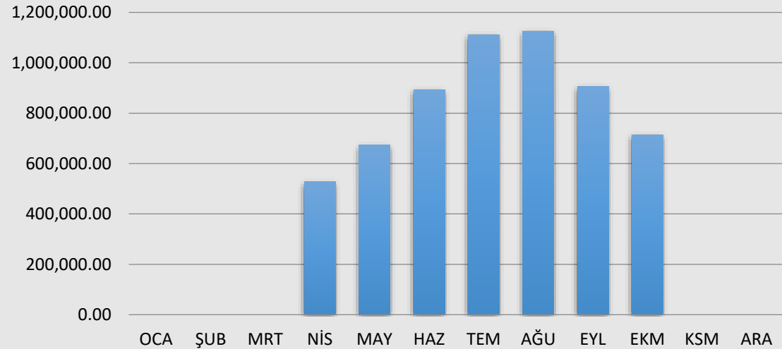
2023 YILI ENERJİ TÜKETİMİ - ELEKTRİK MİKTAR/AY
